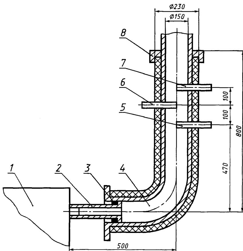
Рисунок 2 — Труба термоизолированная для выполнения измерений
